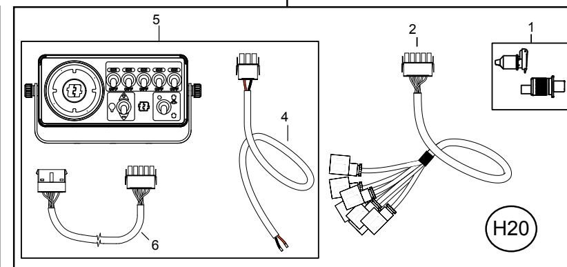
3 Pulsantiera Acqua 5 Vie
