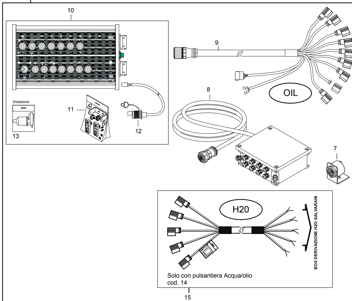
14 Pulsantiera Acqua 5 vie / olio 7 vie
